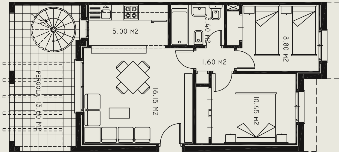
PLANTA BAJA
